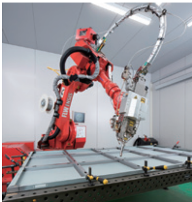
ファイバーレーザ溶接機
