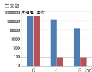
緑膿菌抗菌試験 (JIS R 1702:2012)
